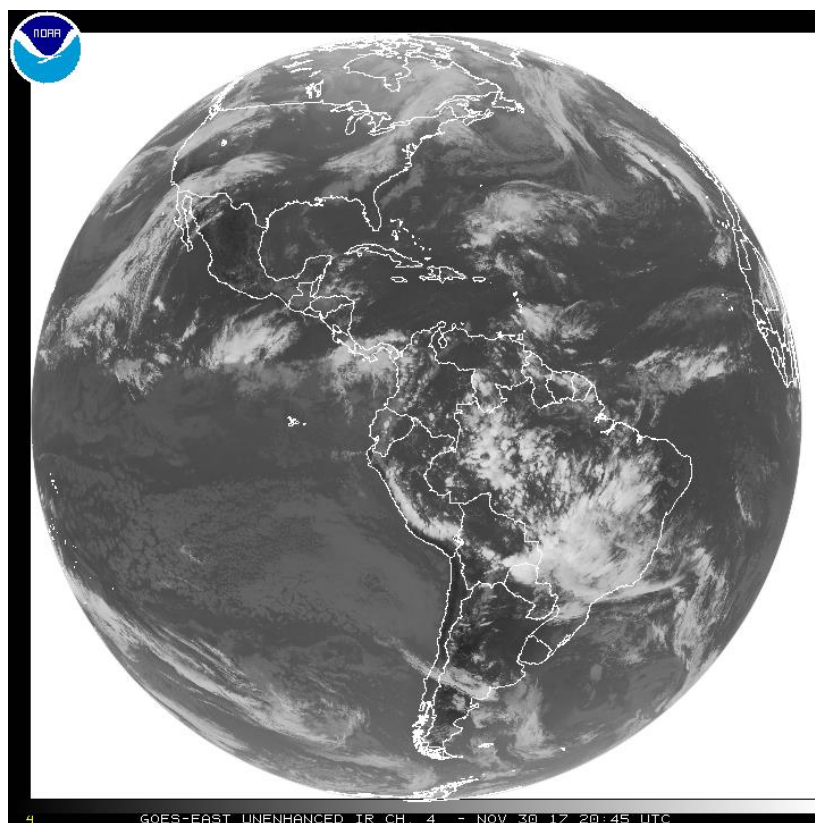
Imagen en el espectro infrarrojo, para el hemisferio occidental, 30 de noviembre de 2017, 3:45 p.m.. Fuente: NOAA
