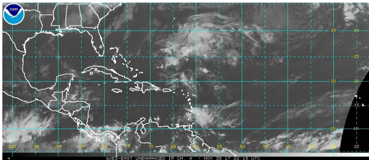
Imagen en el espectro infrarrojo, para el Atlántico Tropical, 30 de noviembre de 2017 a las 5:15 p.m.. Fuente: NOAA
